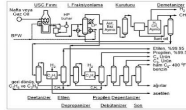
Etilen Üretimi (USC Prosesi)
